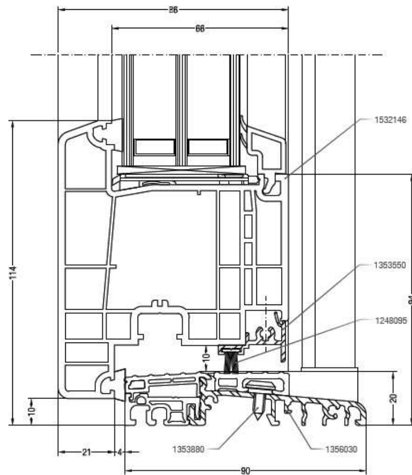
Sezione nodo anta dritta da 117 mm e soglia in Al Apertura esterna
