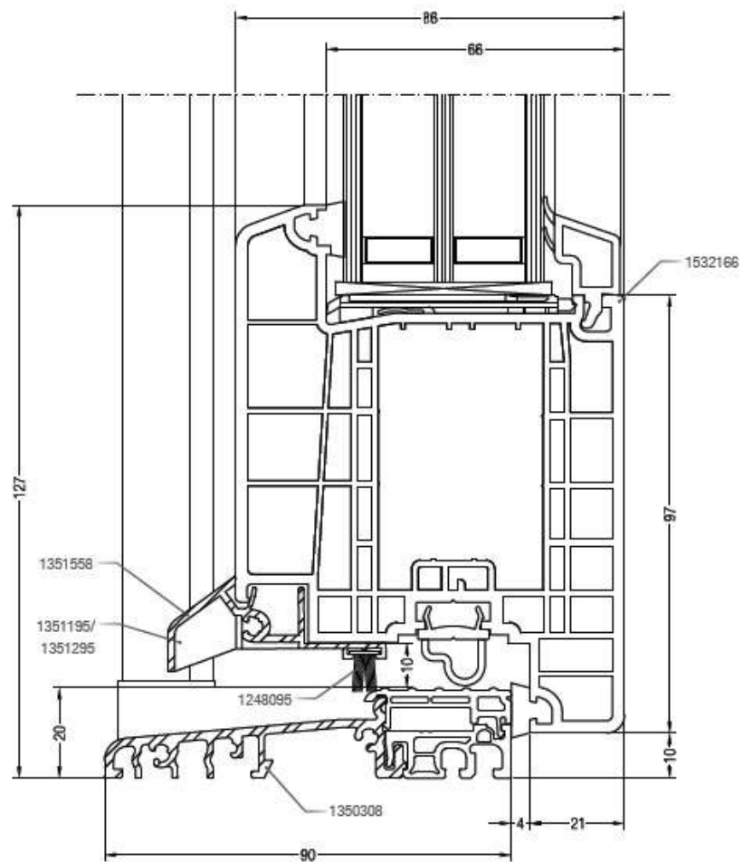
Sezione nodo anta dritta da 97 mm e soglia in Al Apertura interna
